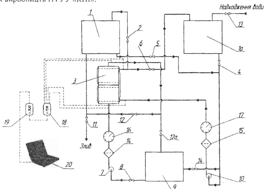
1, 1а – ємності холодної води; 2, 4, 5, 6, 8, 11, 12, 12а, 13 – вентилі; 3 – блочний графітовий теплообмінник; 7, 10 – відцентрові насоси; 9 – ємність гарячої води; 14, 15 – фільтри; 16, 17 – витратоміри; 18 – аналогово-цифровий модуль І-7018; 19 – інтерфейсний модуль І-7520; 20 – ПК.
