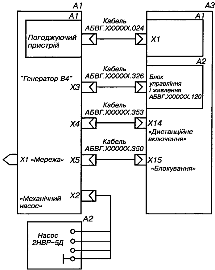
Рис. 8.11 – Схема з'єднань 162
